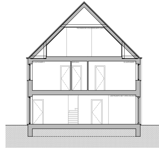
SNEDE
